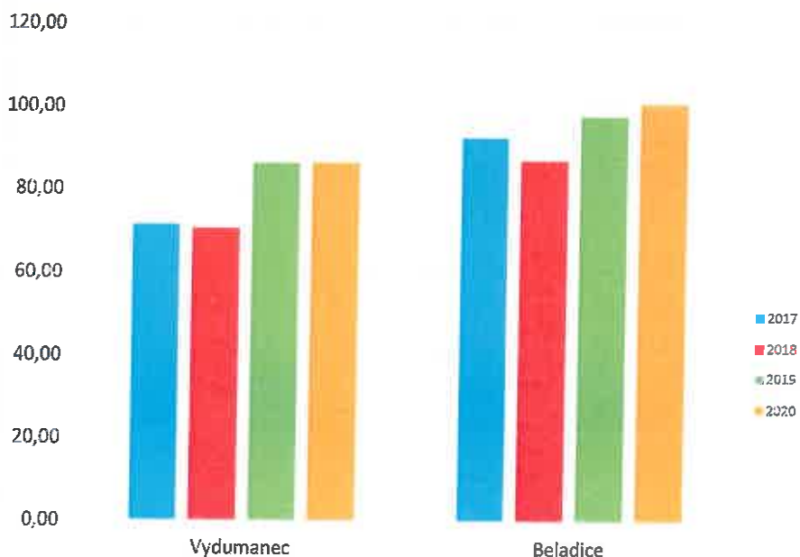
Indikátor IND 2 spotreby energie na obaľovniach v prepócte na 1t vyrobenej zmesi
